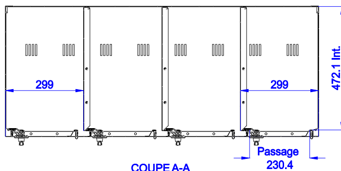
COUPE A-A
