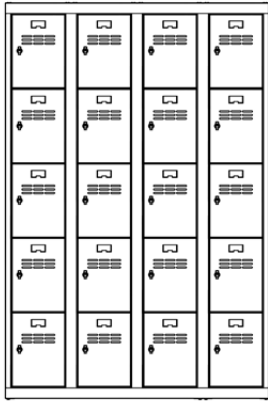
réf. CME534 L.1200 x P.500 x H.1800 mm
