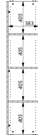
COUPE A-A ECHELLE 1 : 14
