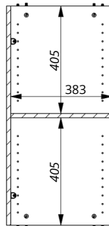
COUPE A-A
