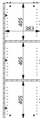
COUPE A-A ECHELLE 1 : 12
